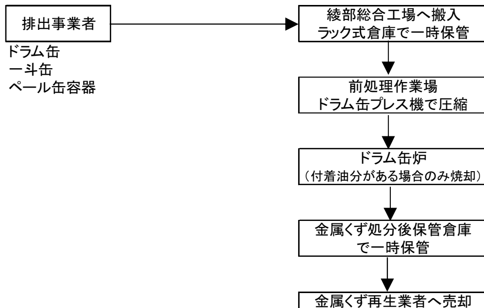
図1.6 処理フロー図（金属くず圧縮施設）（1/2）案
