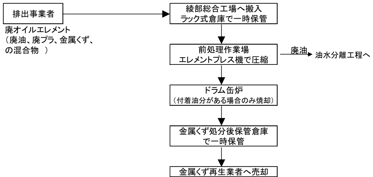
図1.7 処理フロー図（金属くず圧縮施設）（2/2）案
