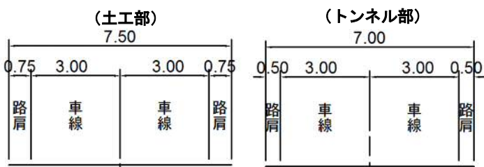
標準断面図
