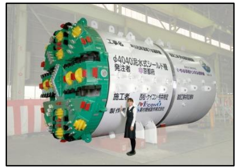
シールド掘削機 (外径 4.04m)
