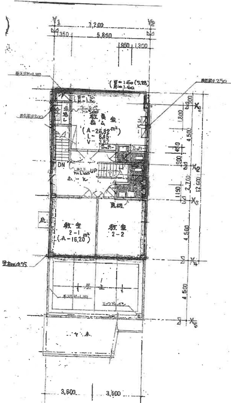
2 階 面 積 1/100 A 2 - 89.51 m 2
