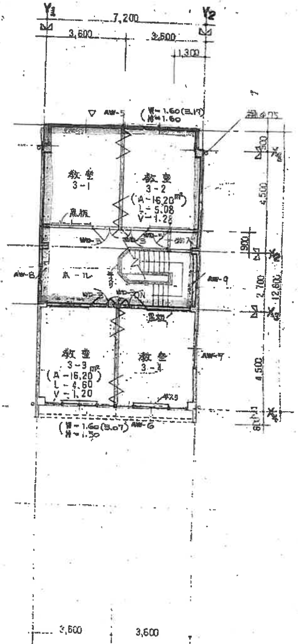
3 階 面 積 1/100 A 3 - 90.72 m 2
