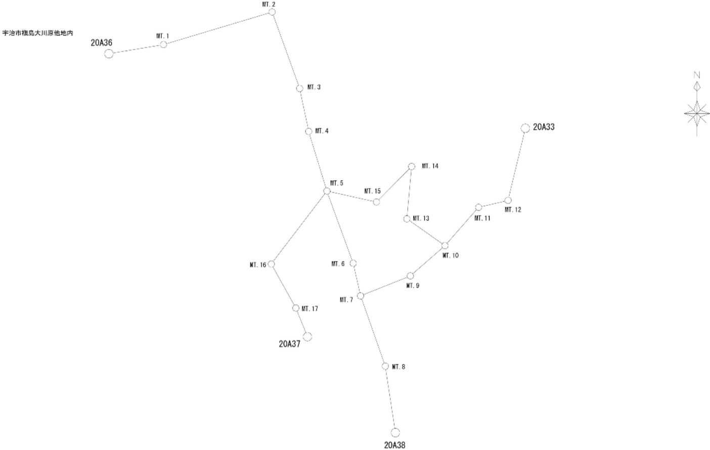
4 級基準点網図
