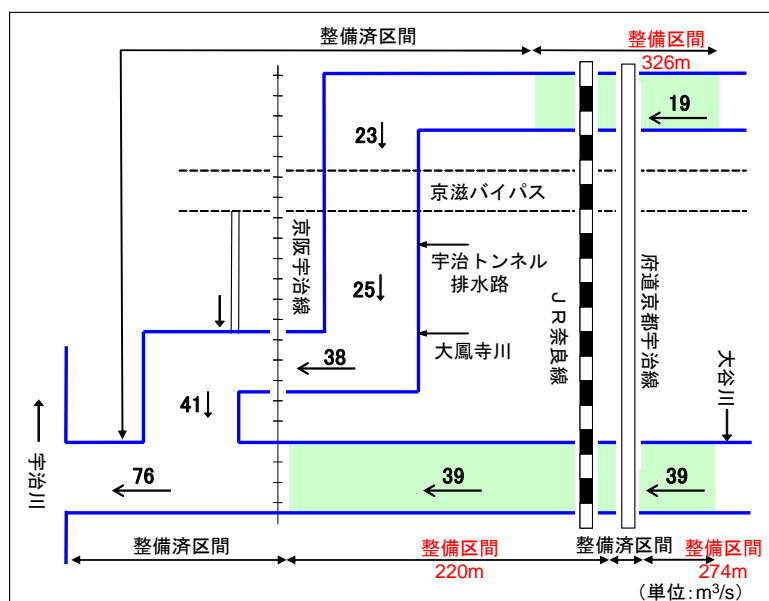
図 2-20 戦川・新田川計画流量配分図 (1/50 規模)
