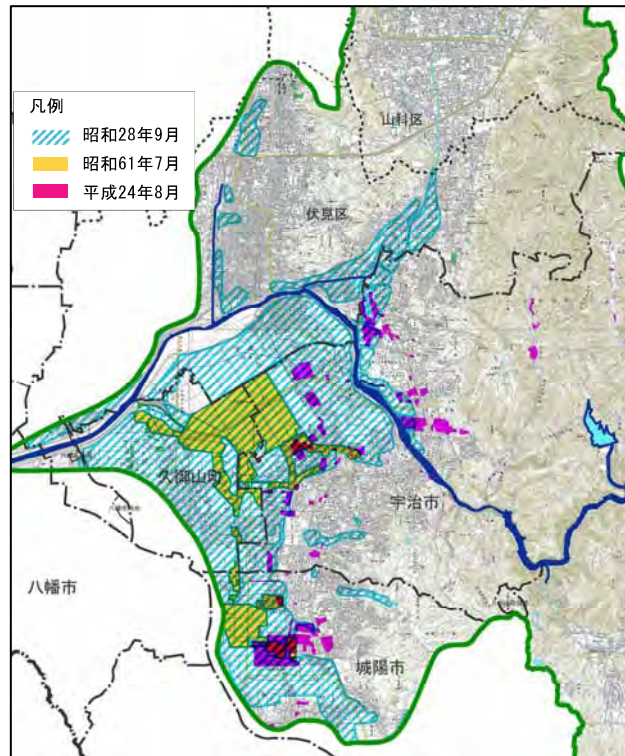
図 1-6 主要洪水の浸水域
