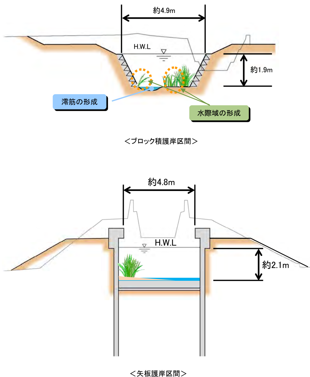
図 2-18 弥陀次郎川標準横断面図
