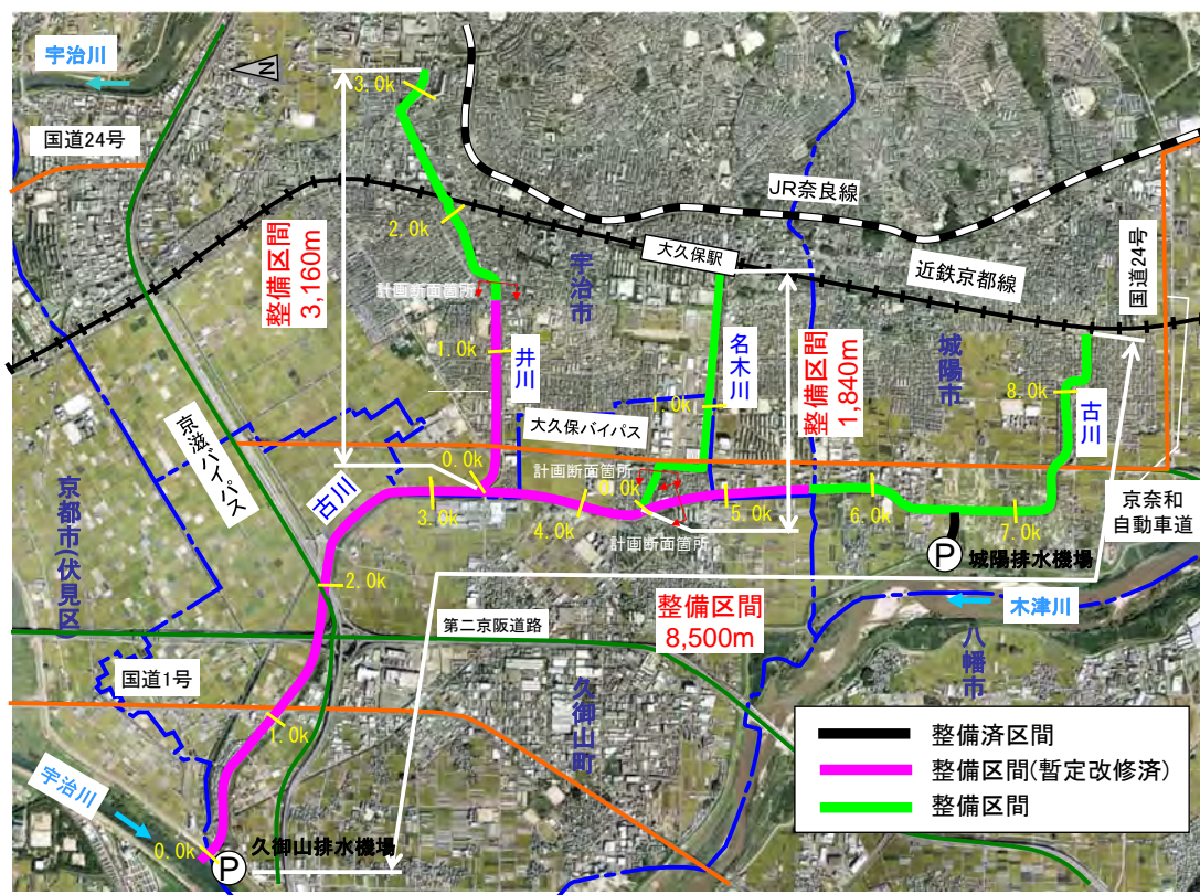
図 2-1 古川、井川、名木川の整備区間
