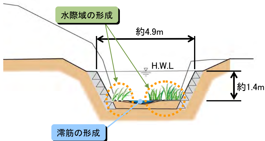
図 2-9 七瀬川標準横断図
