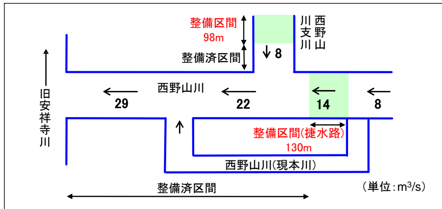
図 2-14 西野山川・西野山川支川計画流量配分図 (1/10 規模)
