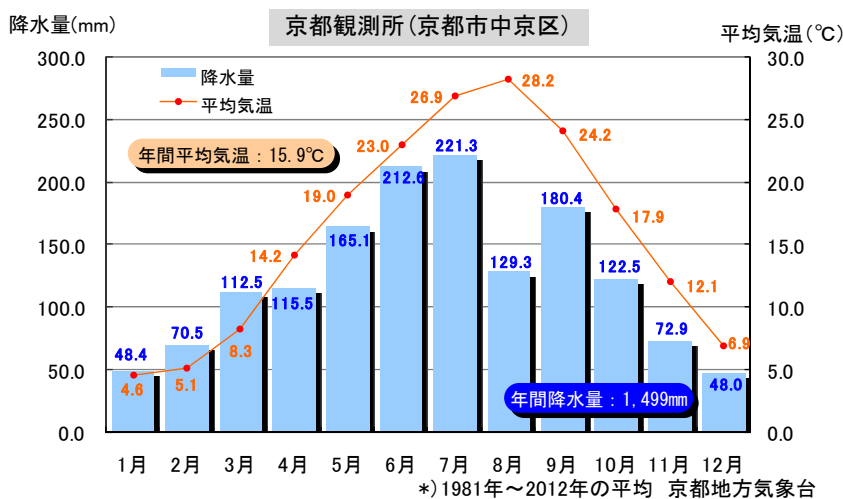
図 1-3 気温と降水量
