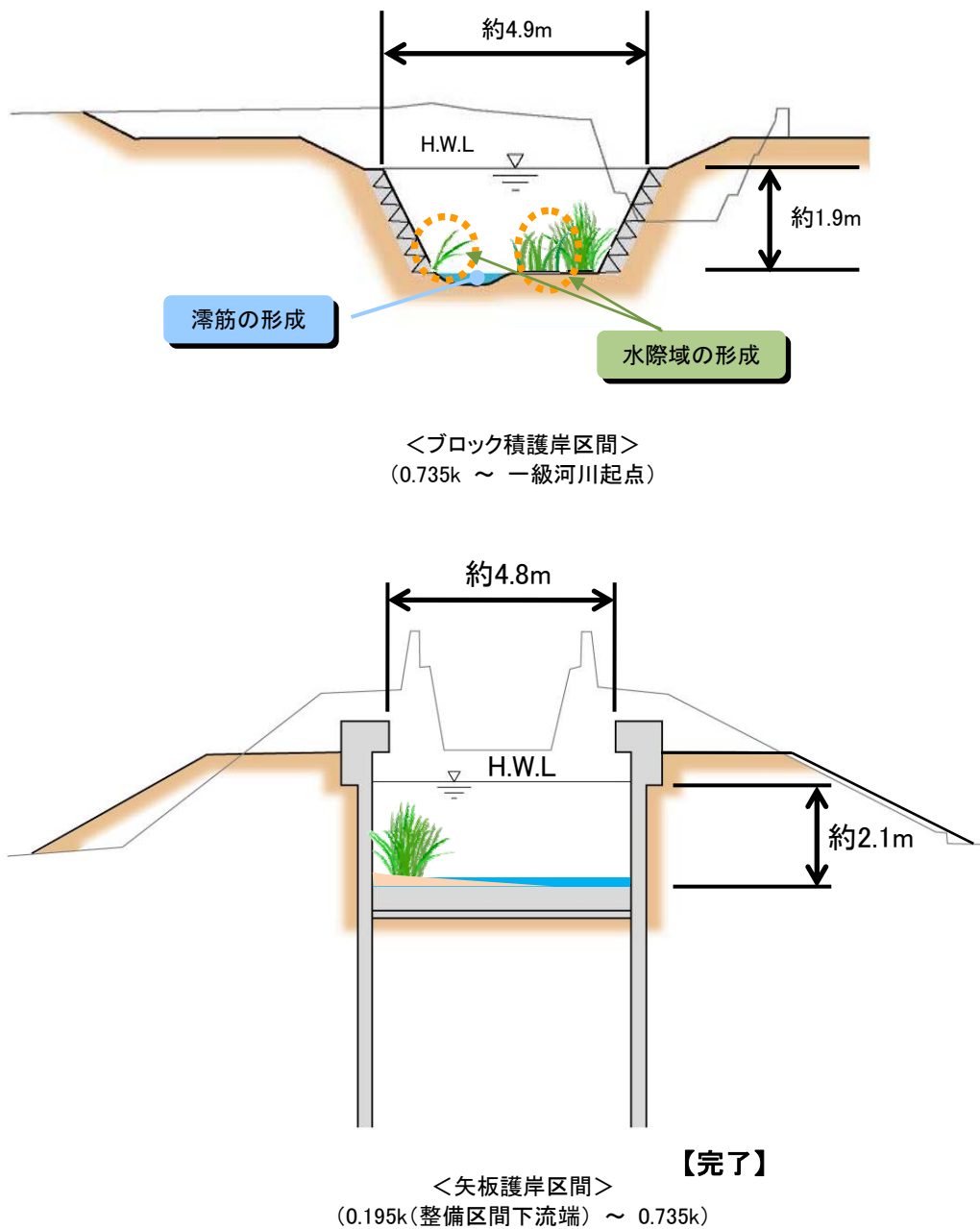
図 2-18 弥陀次郎川標準横断面
