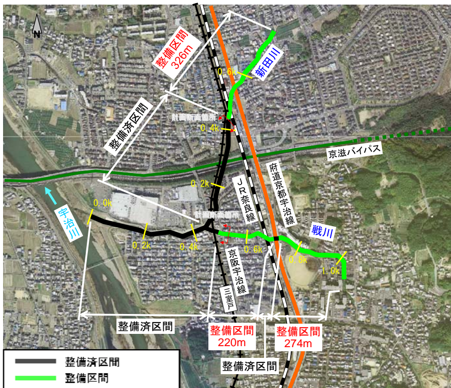
図 2-19 戦川・新田川の実備区間
