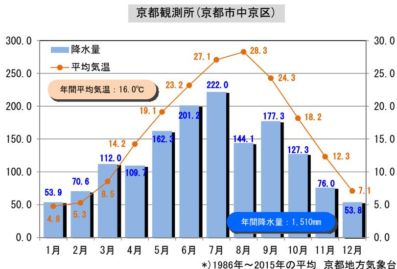
図 1-3 気温と降水量
