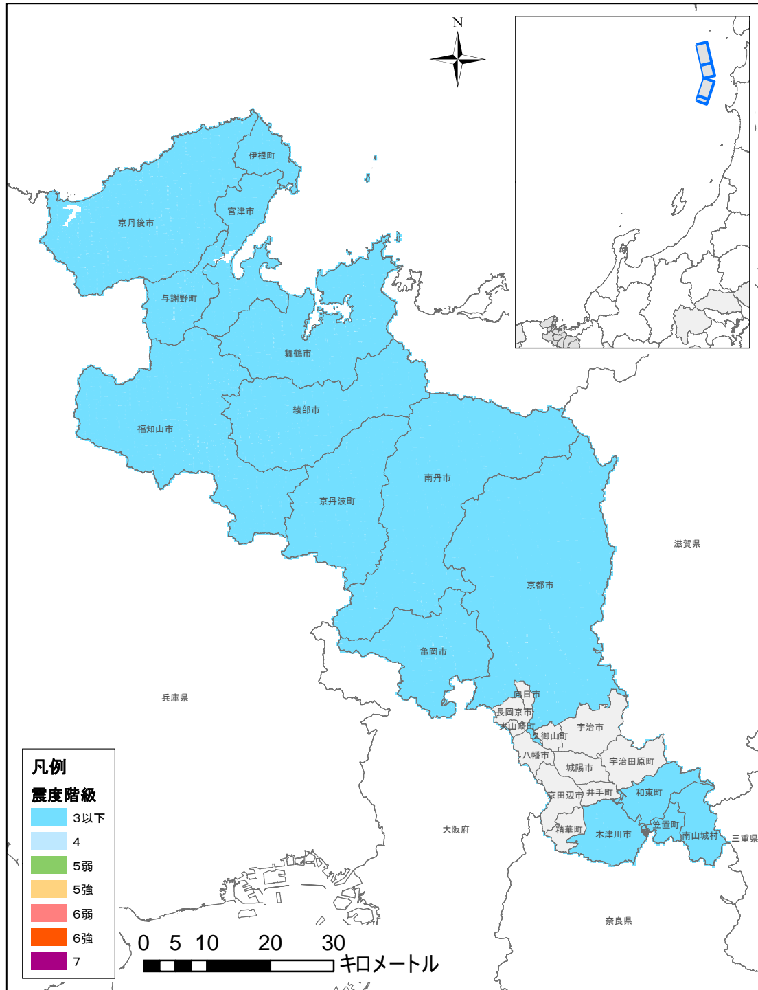
図 2(1)② 震度分布図 (F24) (グリーン関数+距離減衰)
