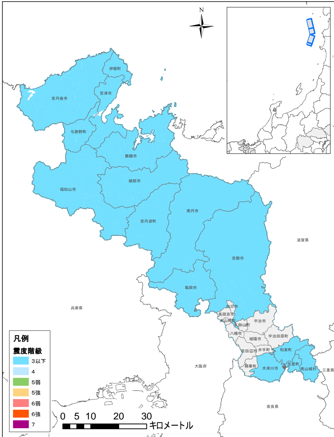
図 2(2)② 震度分布図 (F24) (グリーン関数+距離減衰)
