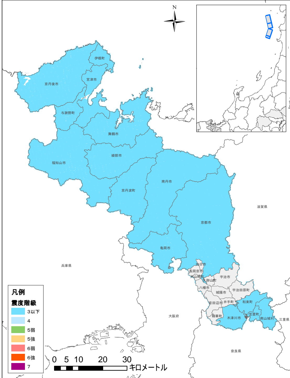
図 2(4)② 震度分布図 (F24) (グリーン関数+距離減衰)
