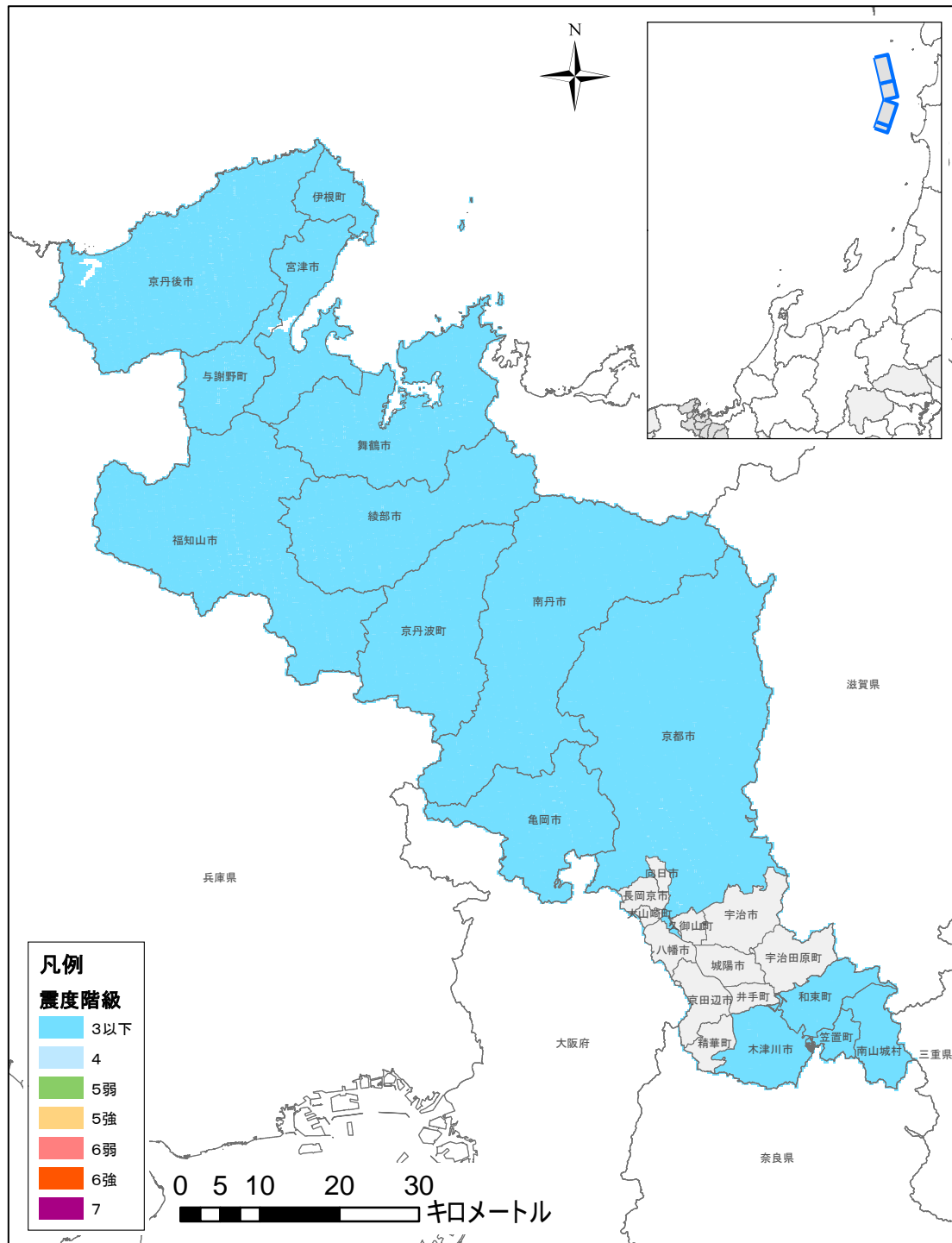
図 2(4)① 震度分布図 (F24) (グリーン関数)
