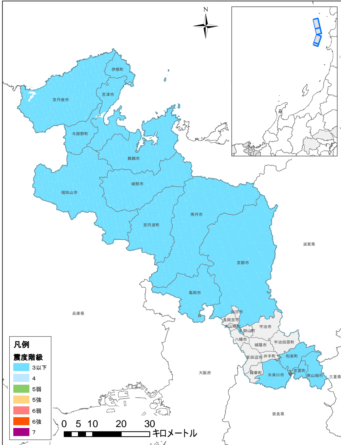
図 2(3)① 震度分布図 (F24) (グリーン関数)
