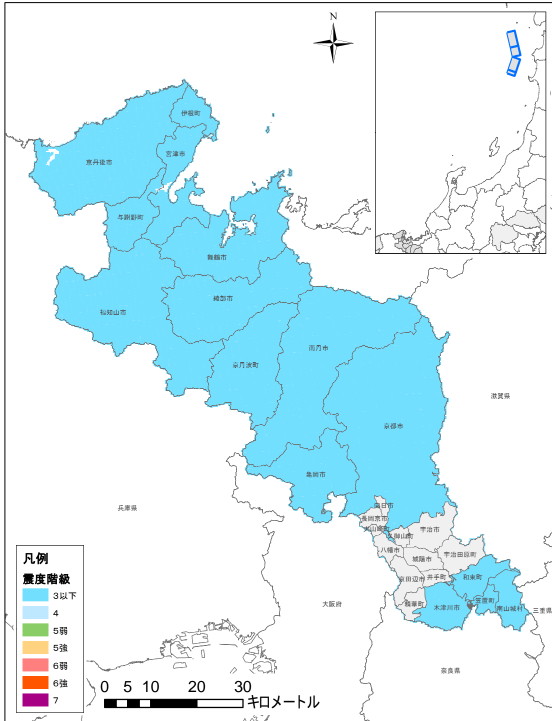
図 2(2)① 震度分布図 (F24) (グリーン関数)
