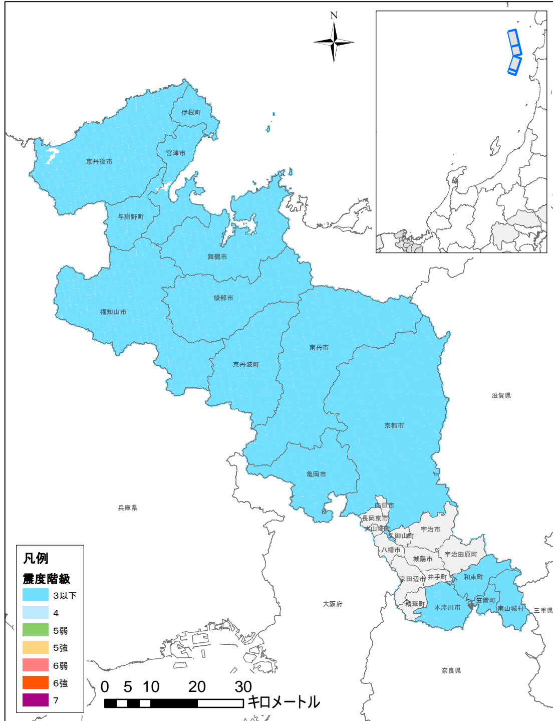
図 2(1)① 震度分布図 (F24) (グリーン関数)
