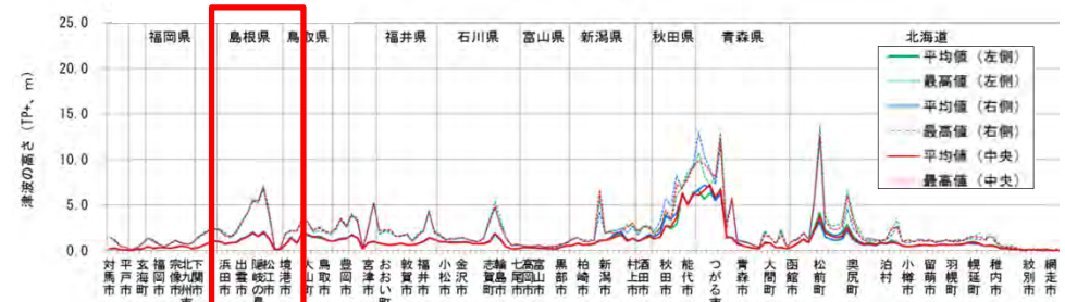
市町村別の平均津波高および最大津波高(F24)
