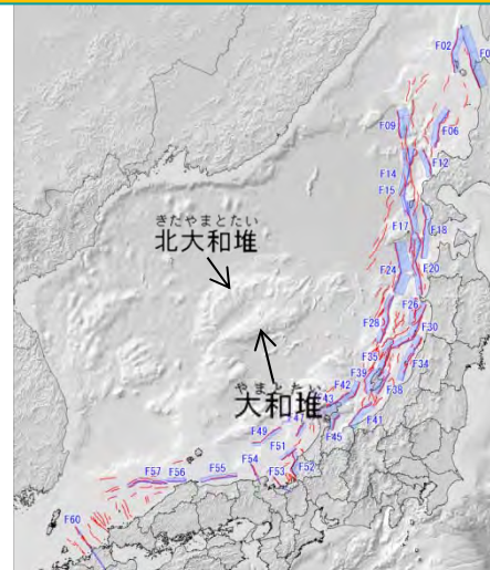
日本海の海底地形
