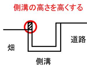
横断図
