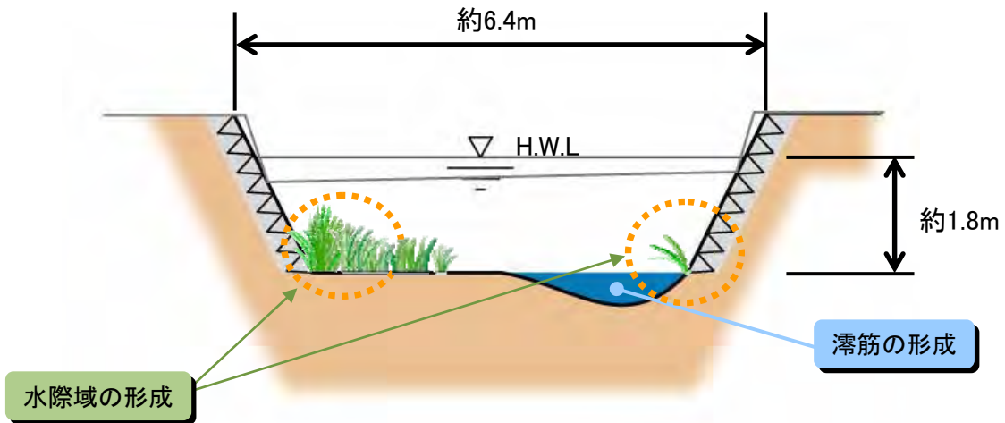
図 2-6 東高瀬川標準横断面図
