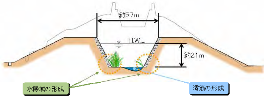
図 2-18 弥陀次郎川標準横断面図
