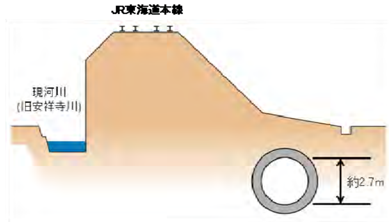
図 2-12 旧安祥寺川標準横断面
