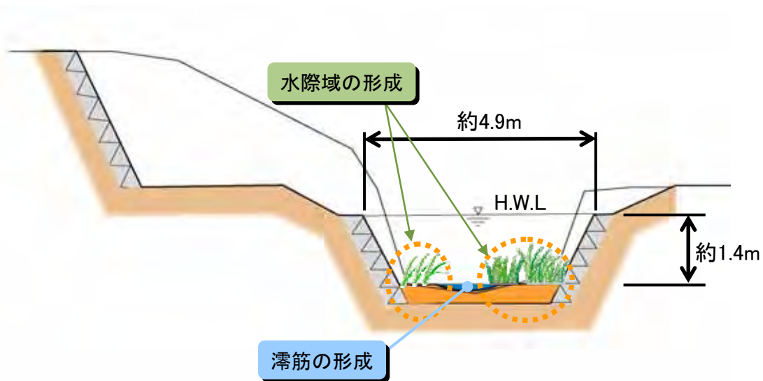
図 2-9 七瀬川標準横断面図
