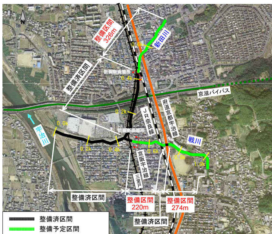
図 2-19 戦川・新田川の間整備区間
