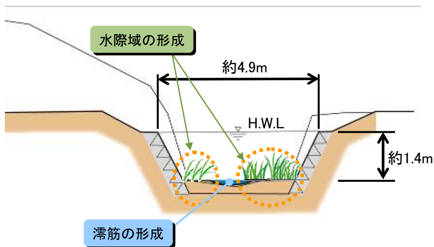
図 2-9 七瀬川標準横断面図
