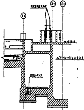
断面 F-F
