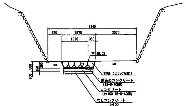
構造図
