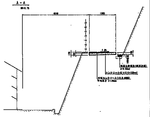
構造図 S=1:20
