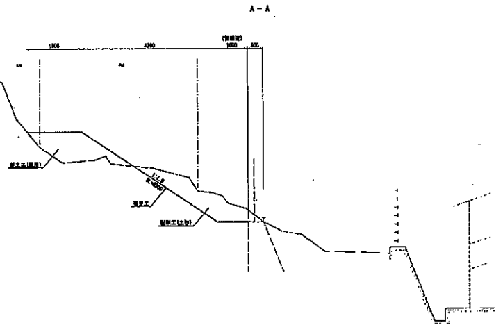
標準横断面図 S=1:50
