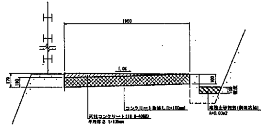
(天端コンクリート修繕 標準横断面図)
