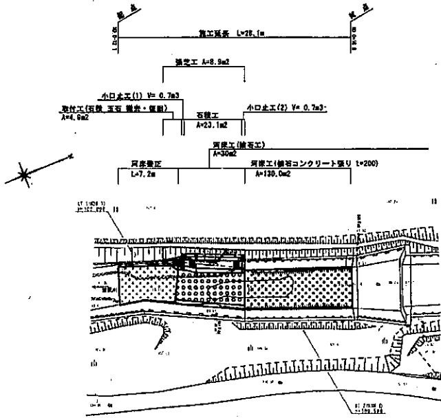
波見川 計画平面図 S=1:250
