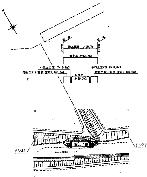
波見川 計画平面図 S=1:250
