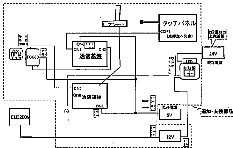
電気系統図
