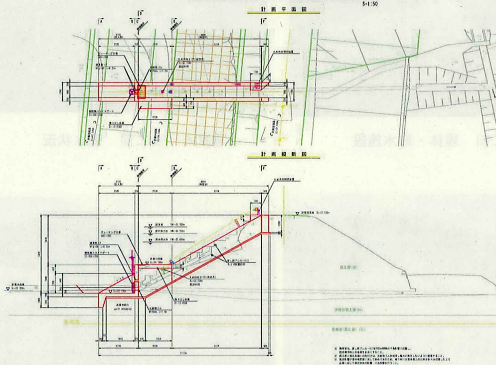
取水施設構造圖 (1/2)
