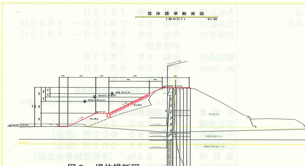
図3 堤体横断面図
