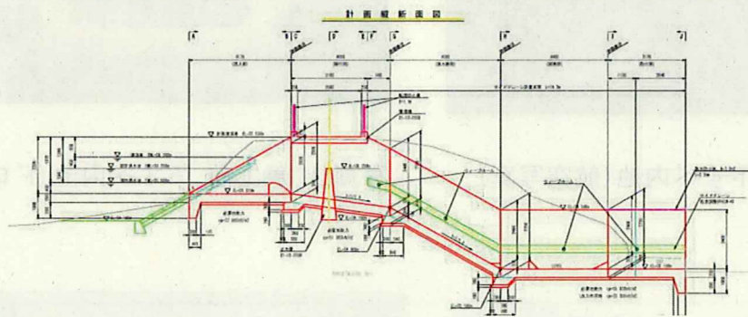
圖 4 洪水吐構造圖
