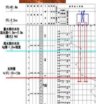
図-4-2 杭基礎図
