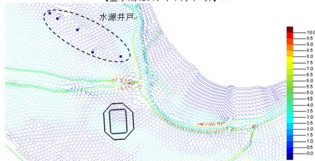
図-5-2 現況の地下水位再現計算結果 (ステップ1のAg層の流速ベクトル、単位：m/d)
