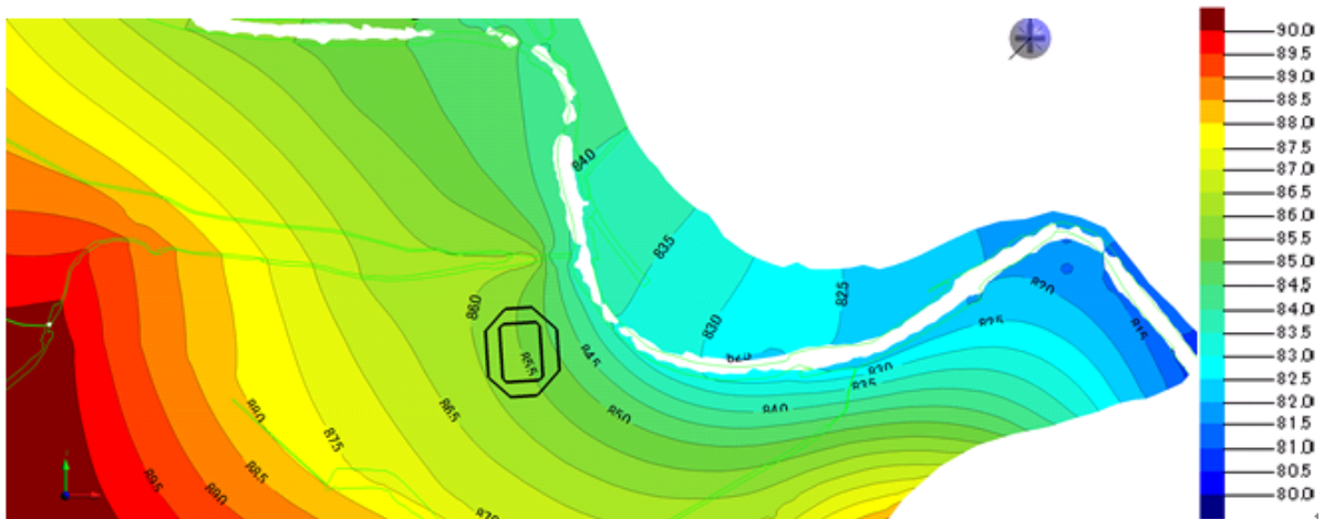
図-5-1 現況の地下水位再現計算結果 (ステップ1の地下水位標高コンター)
