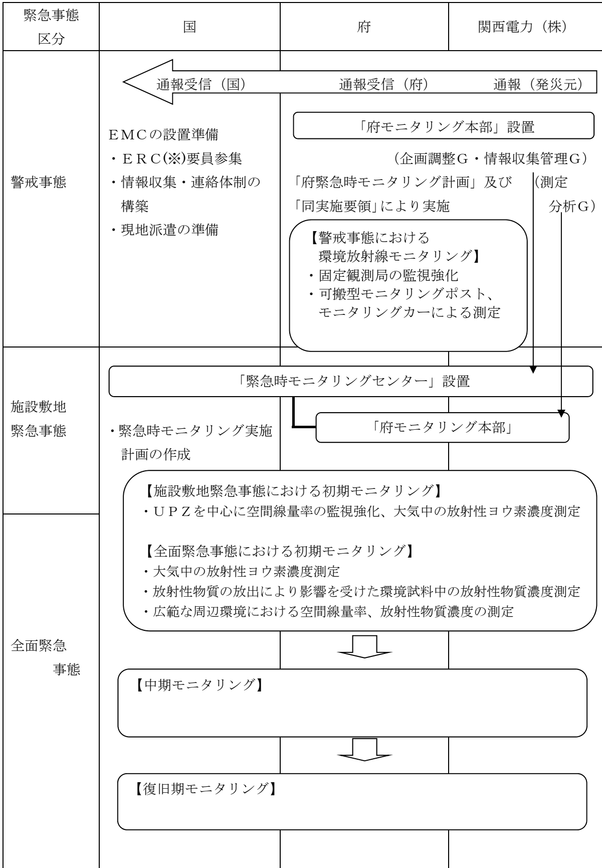
別図1 緊急時モニタリングの実施フロー
