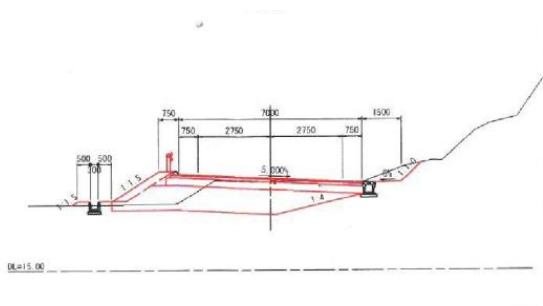
標準断面図
