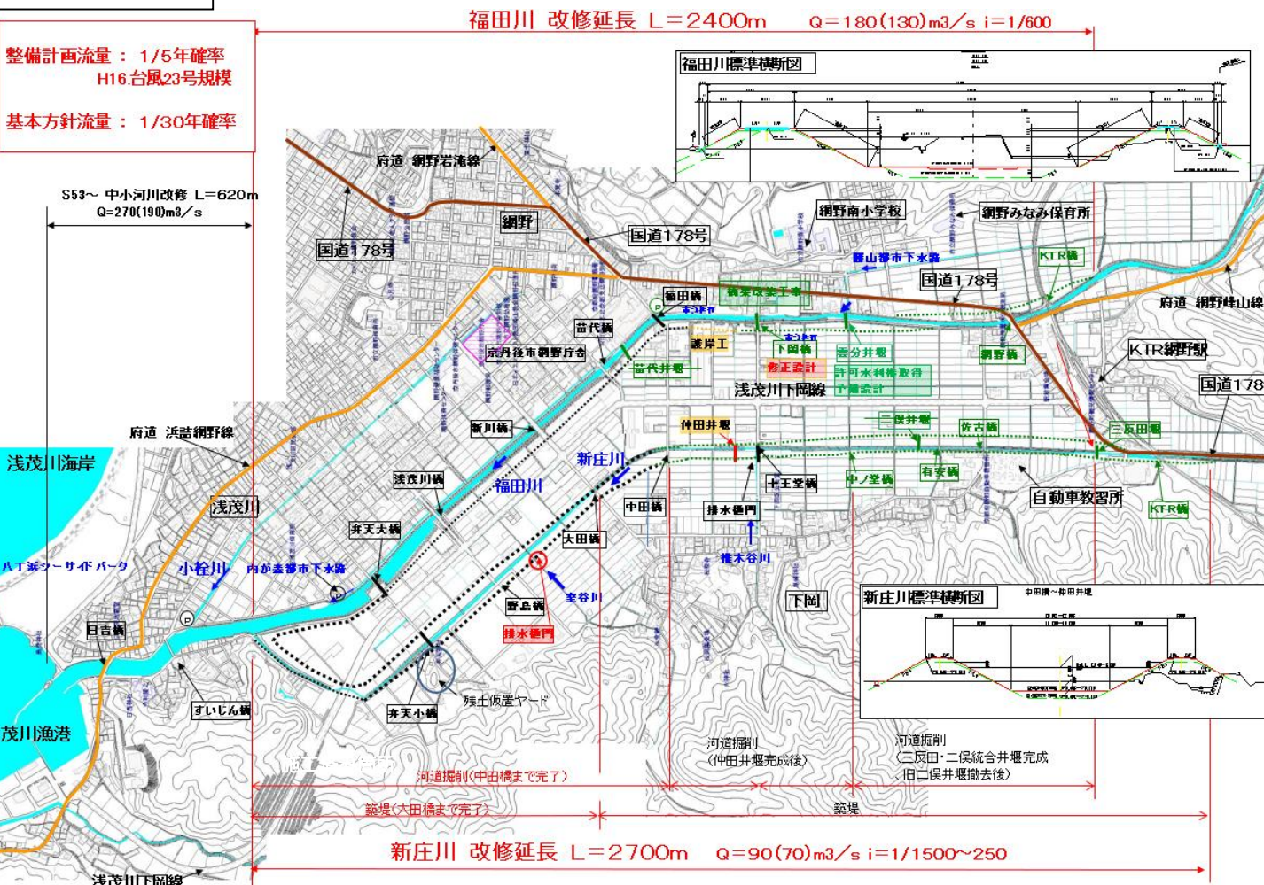
計画平面図
