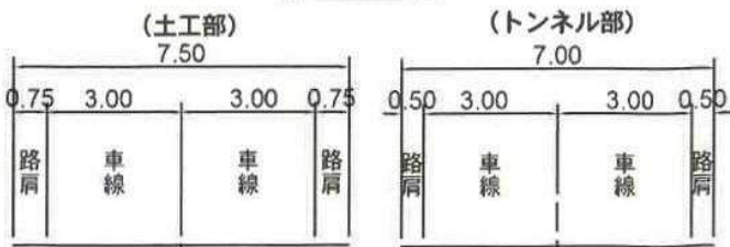
標準断面図
