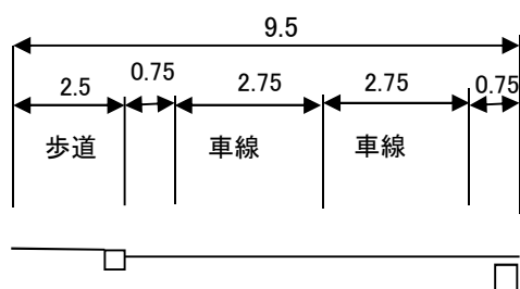
現況幅員5.0m⇒計画幅員9.5m
