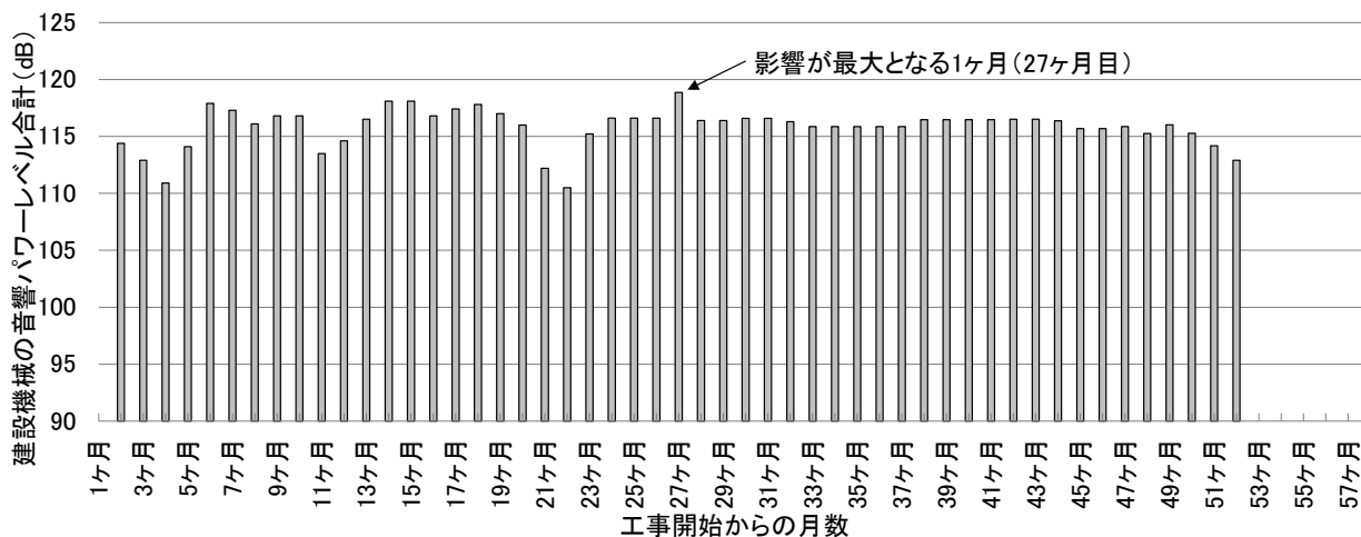
図 7-1.26 建設機械の稼働による騒音予測対象時期
