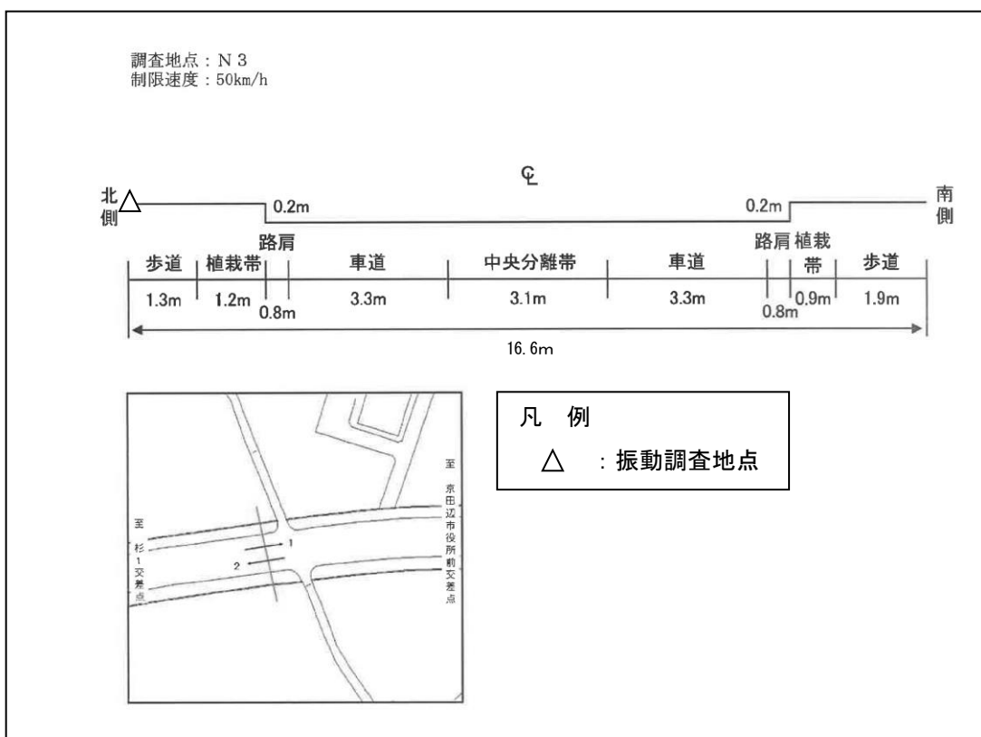
図 7-1.39 道路断面図
