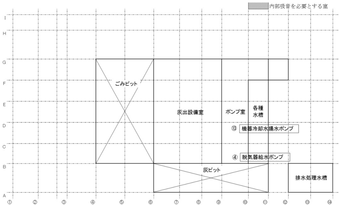
図 5-1-2.12(1) 騒音発生機器の配置 (B1F)
