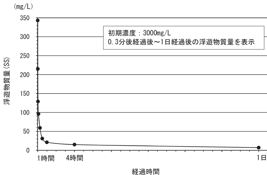
図 5-2.9 経過時間と浮遊物質量(SS)
