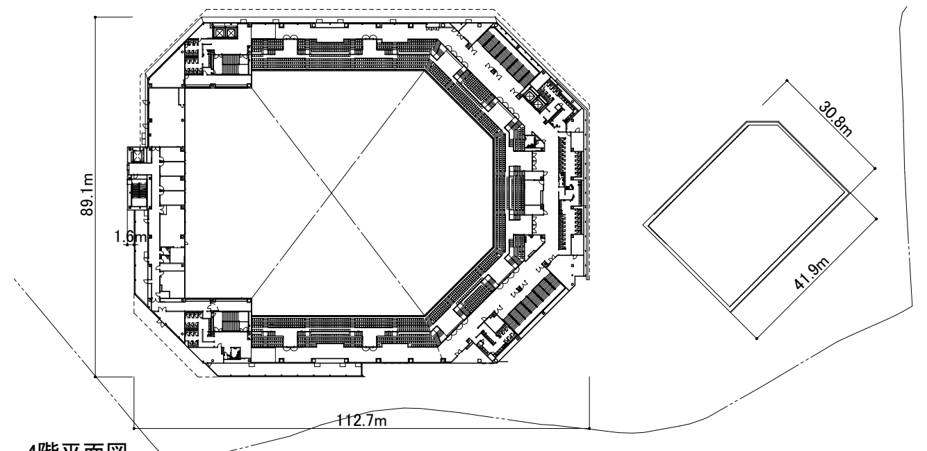
4階平面図
