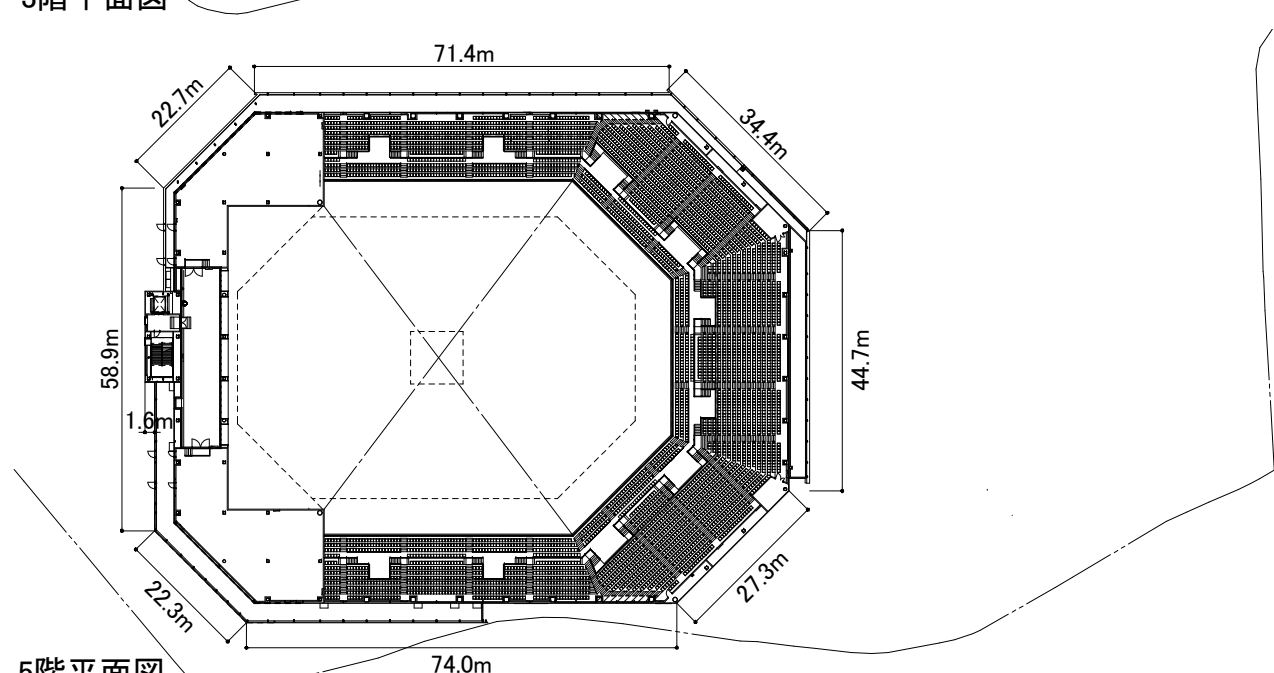
5階平面図
