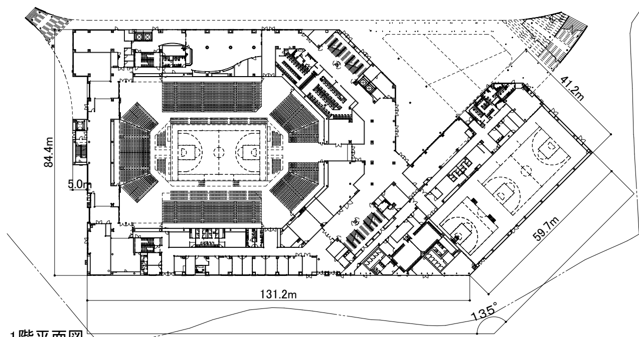
1階平面図
