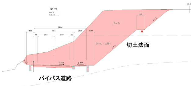
計画断面図
