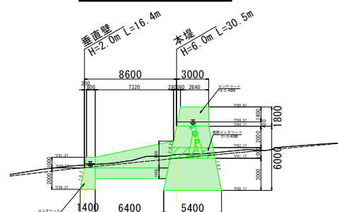
堰堤断面図
