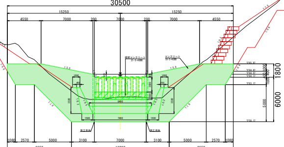
堰堤断面図
