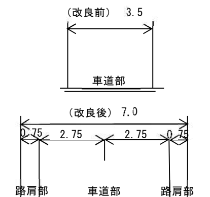
標準横断図 上杉和知線
