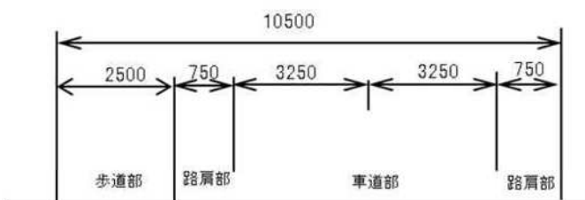
横断図
