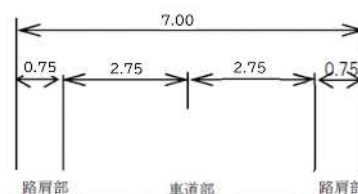
標準断面図 (改良後)
