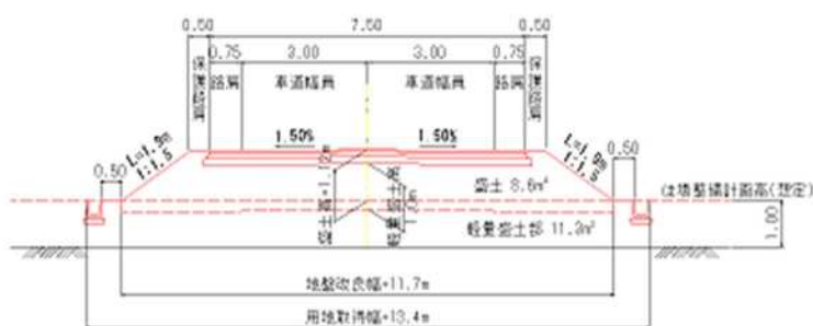
標準断面図 (改良後) バイパス部
