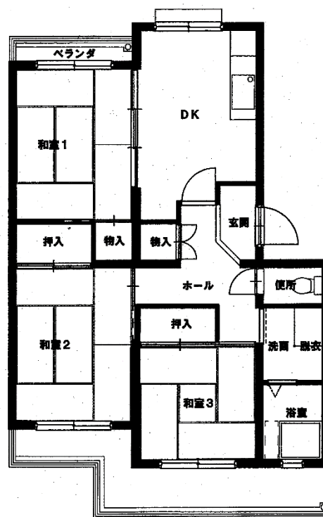
②⑦松蔭団地 3DK（間取図）
