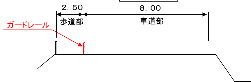
標準断面図
