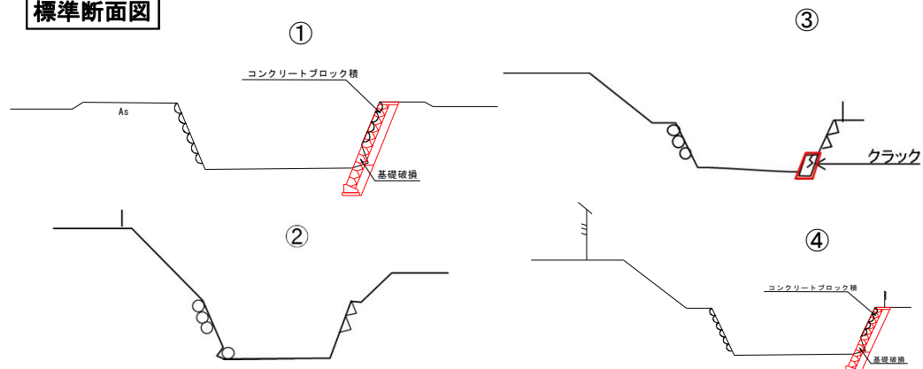
標準断面図
