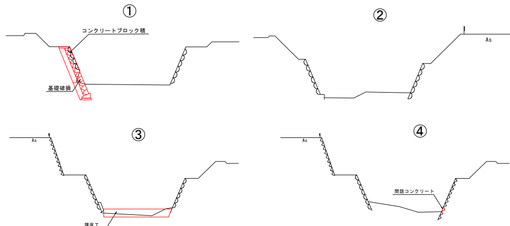
標準断面図
