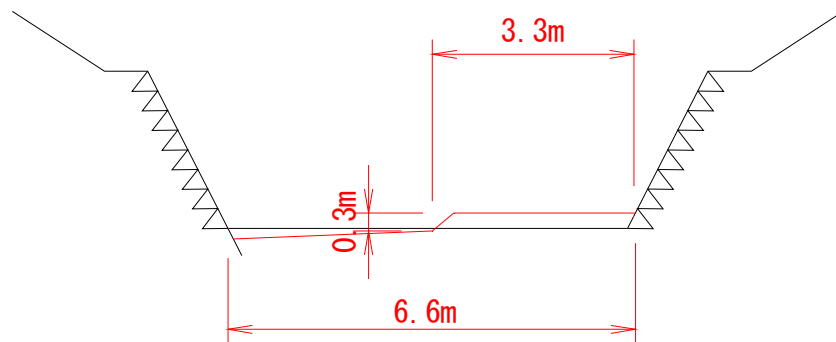
標準断面図
