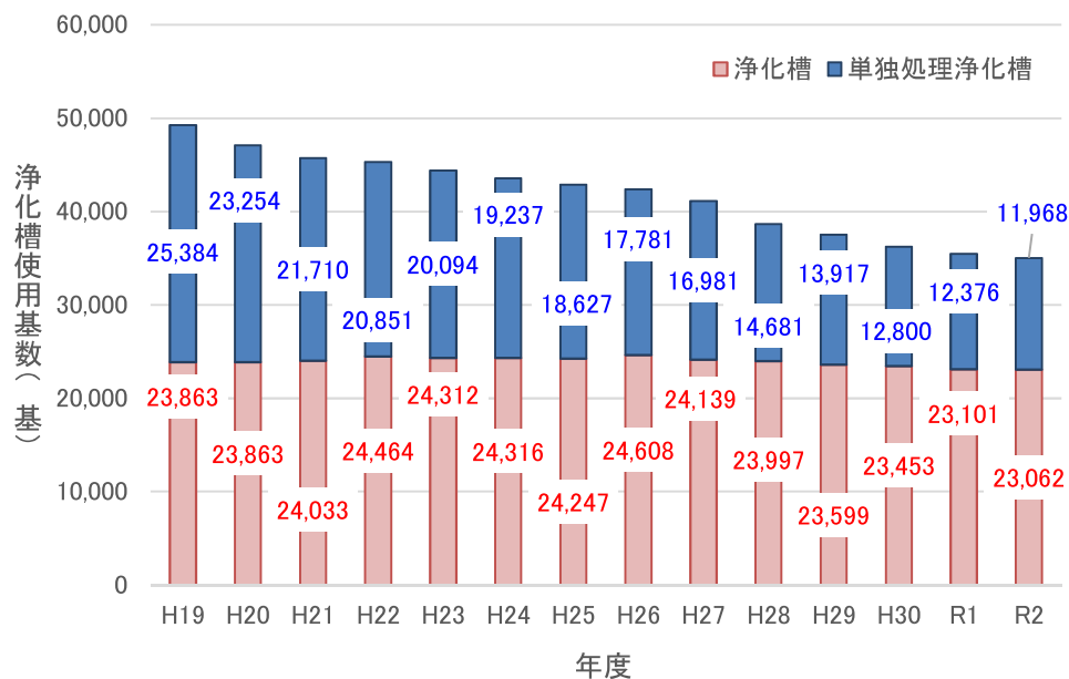
図 11 京都府における浄化槽設置基数
