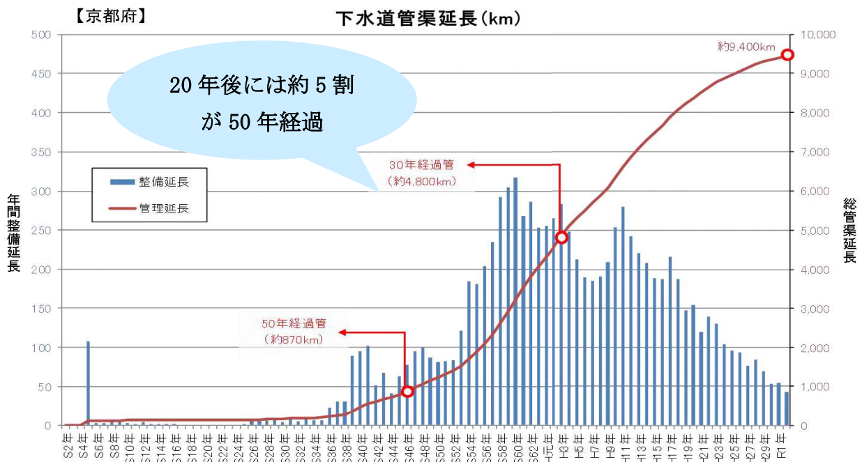
図 16 府内の下水道管渠延長の経年変化
