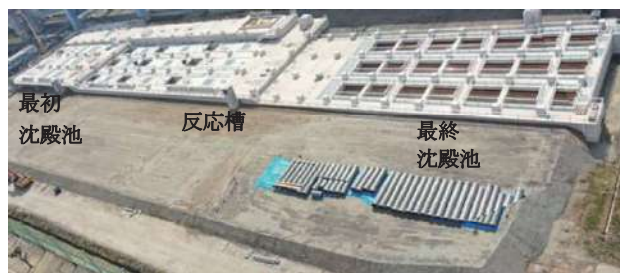
洛南浄化センター水処理施設E1系増設工事（R4年3月時点）
