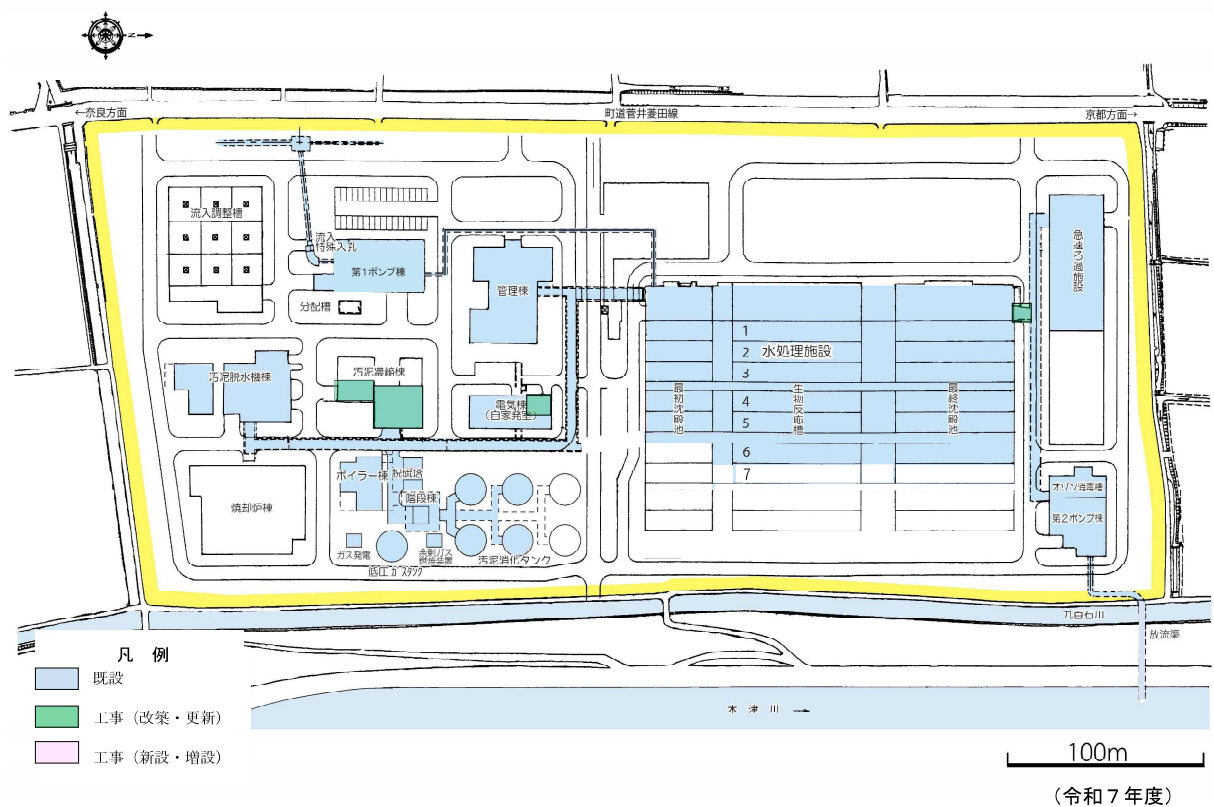
木津川上流浄化センター平面図
