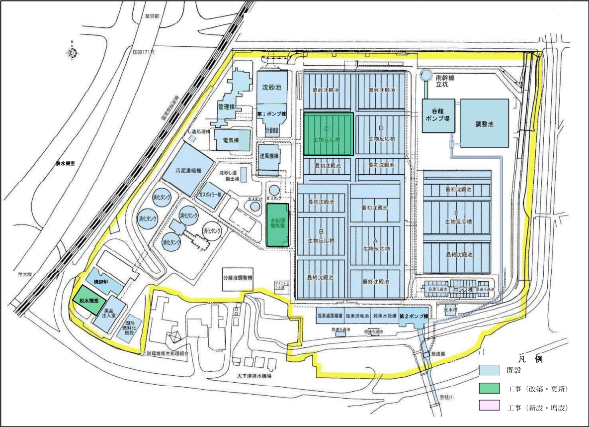
洛西浄化センター平面図
