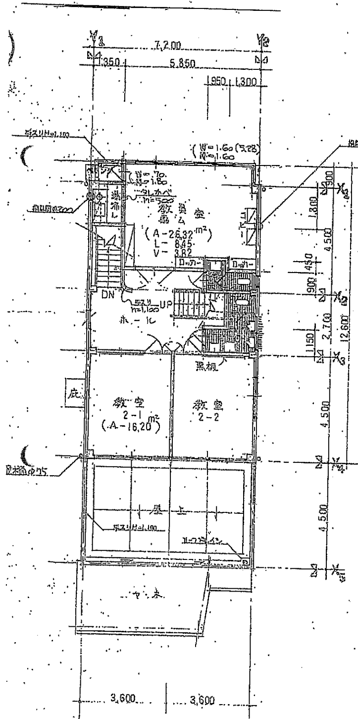
2F平面図 1/100 A 2 = 89.51 m 2
