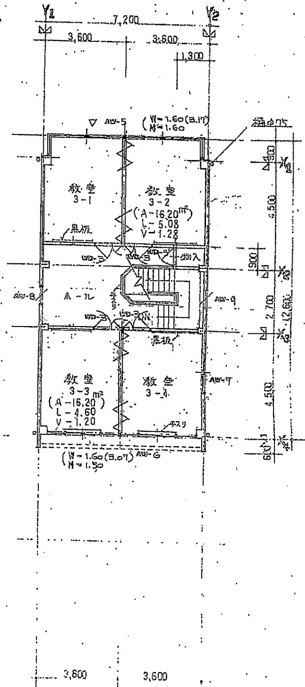
3F平面図 1/100 A 3 = 90.72 m 2
