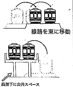
連続立体交差 仮線方式の場合
