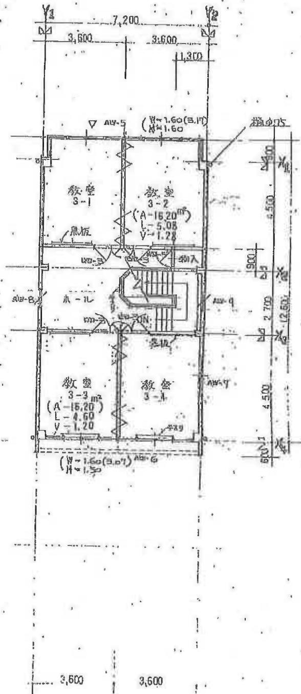
3階平面図 1/100 A 3 = 90.72 m 2
