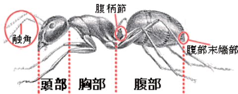
図：アリの体について（アリの王国（ポプラ社学習文庫）クロオオアリ図を一部改変）
