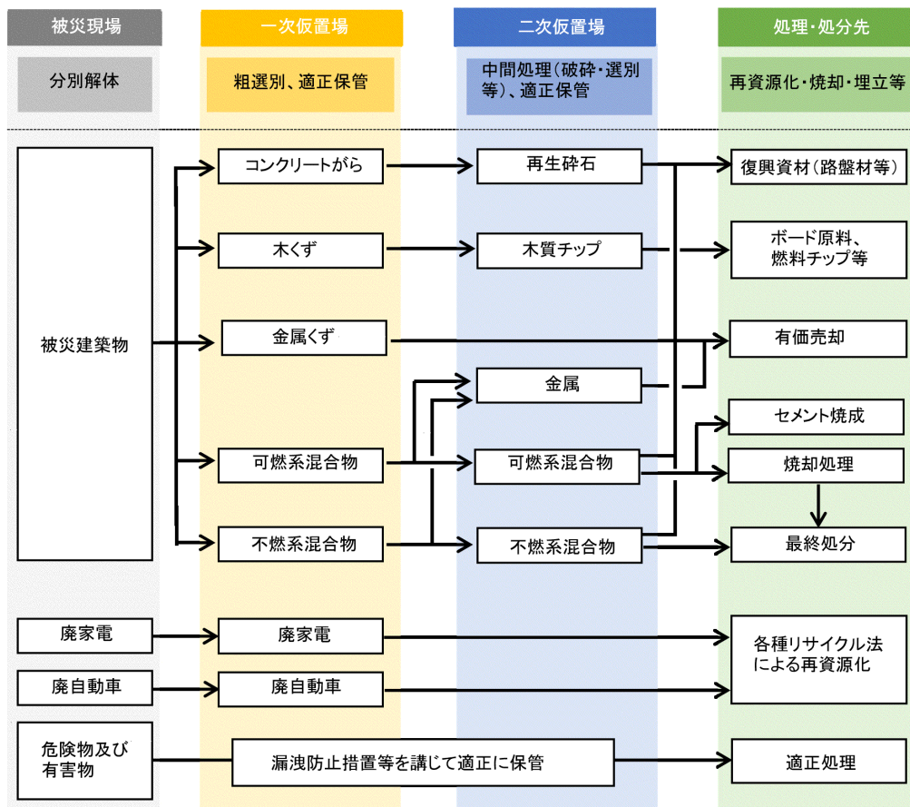
図 4 災害廃棄物の標準処理フロー
