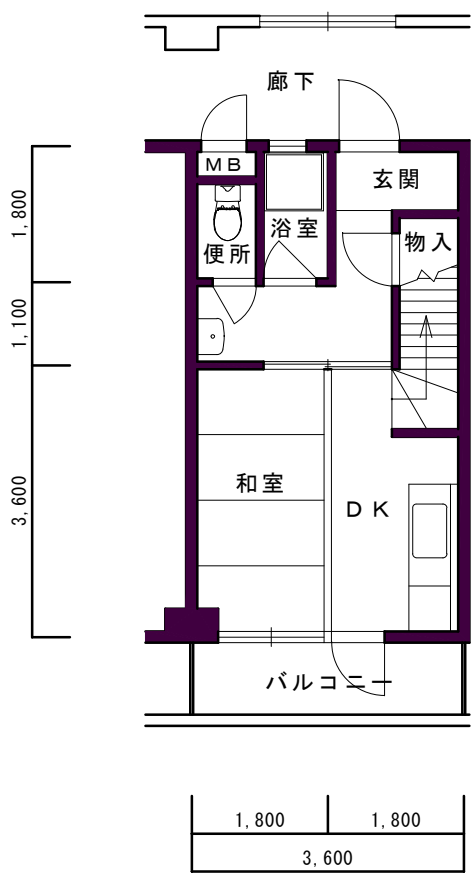
2 , 4 F 間取図
