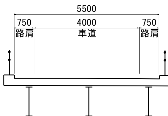
【現況横断面図】
