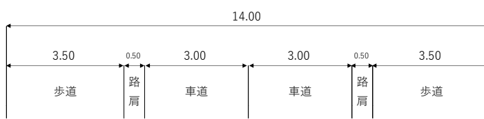
【計画横断面図】
