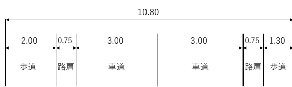
【現況横断面図】
