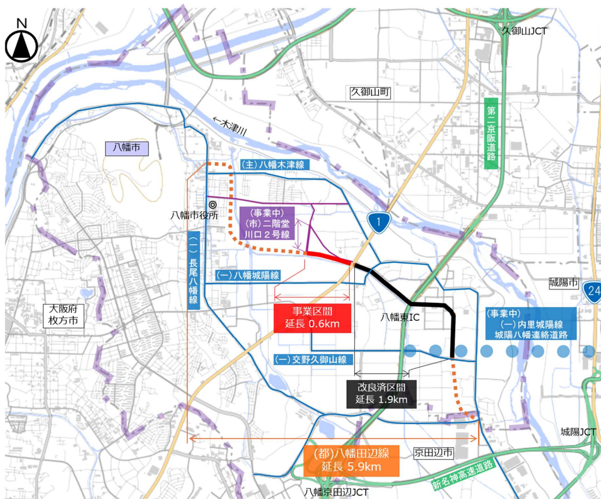
図-3 事業概要図
