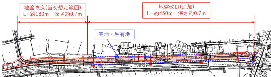
図-10 地盤改良平面図
