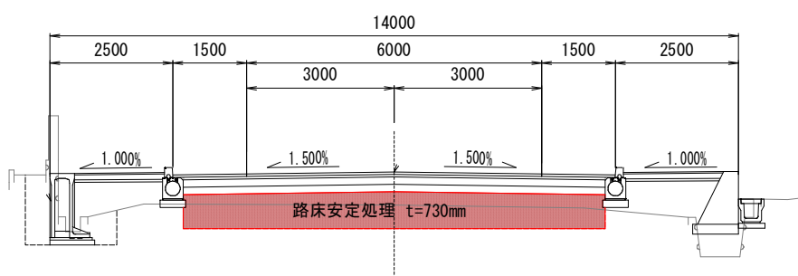
図-11 地盤改良標準横断図
