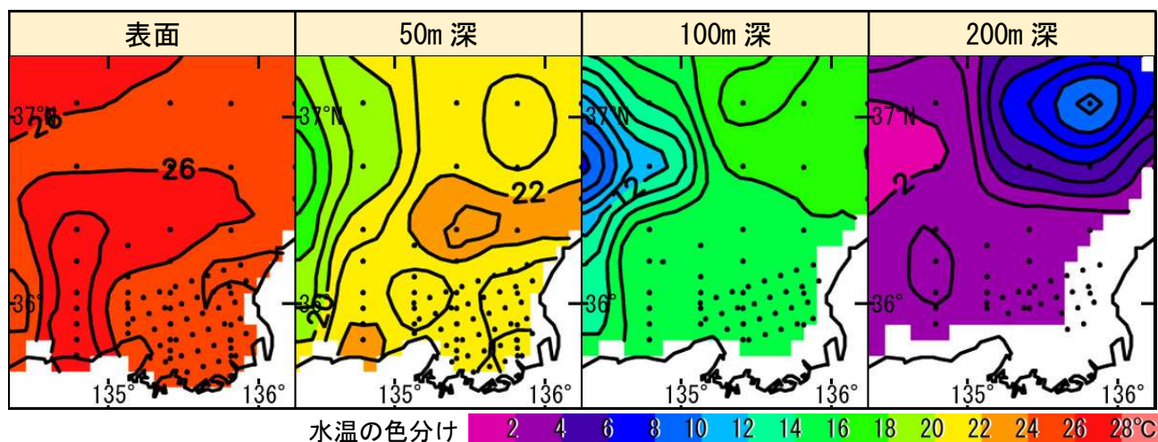
京都府周辺の各層水温(2025 年 10 月上旬)
