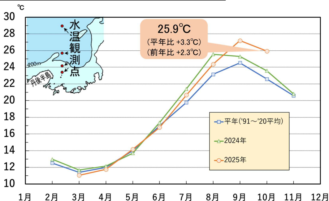
京都府周辺の各層水温(2025 年 10 月上旬)
