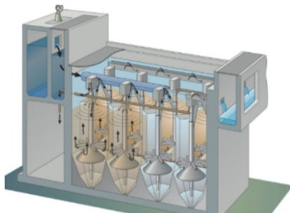
急ろ施設の完成イメージ（能力増強）
